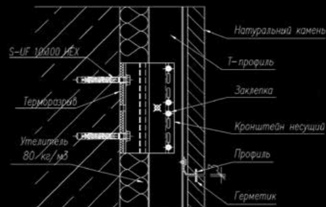
Вертикальное сечение фасада Крепление натурального камня
