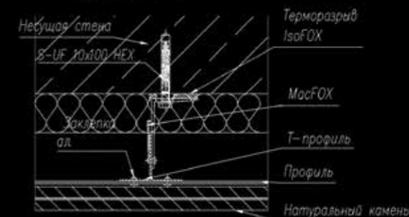
Горизонтальное сечение фасада Рядовой участок
