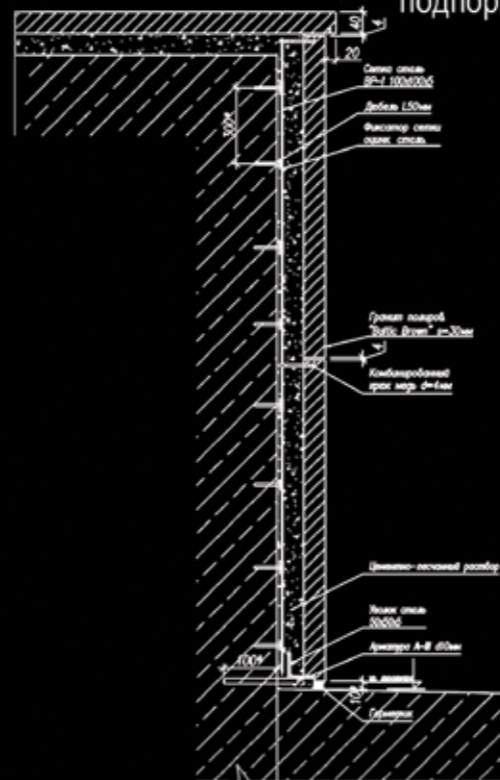
Вертикальное сечение подпорной стены
