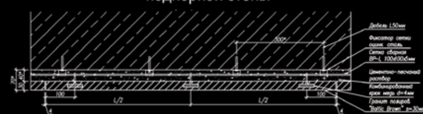
Горизонтальное сечение подпорной стены
